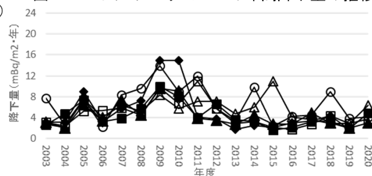
図3-3 プルトニウム-239の年間降下量の推移
