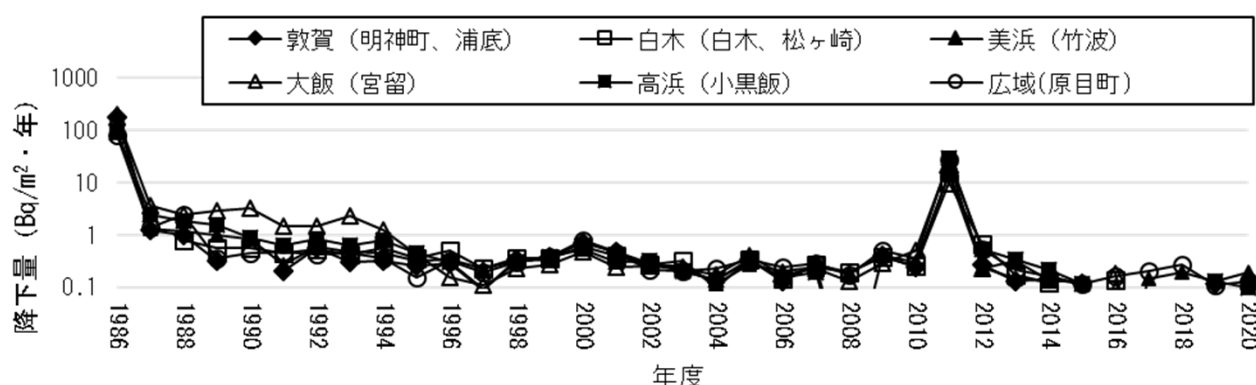
図3-2 ストロンチウム-90の年間降下量の推移
