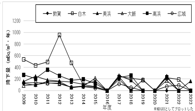
図2-4 ストロンチウム-90の年間降下量の推移
