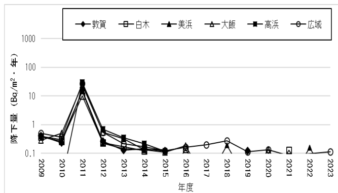
図2-3 セシウム-137の年間降下量の推移
