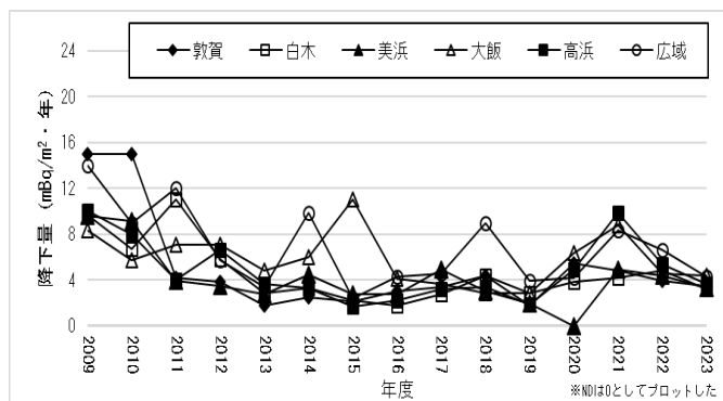
図2-5 プルトニウム-239の年間降下量の推移
