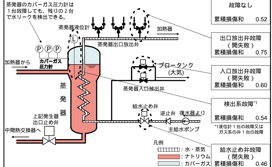
プラント条件の影響評価説明図
