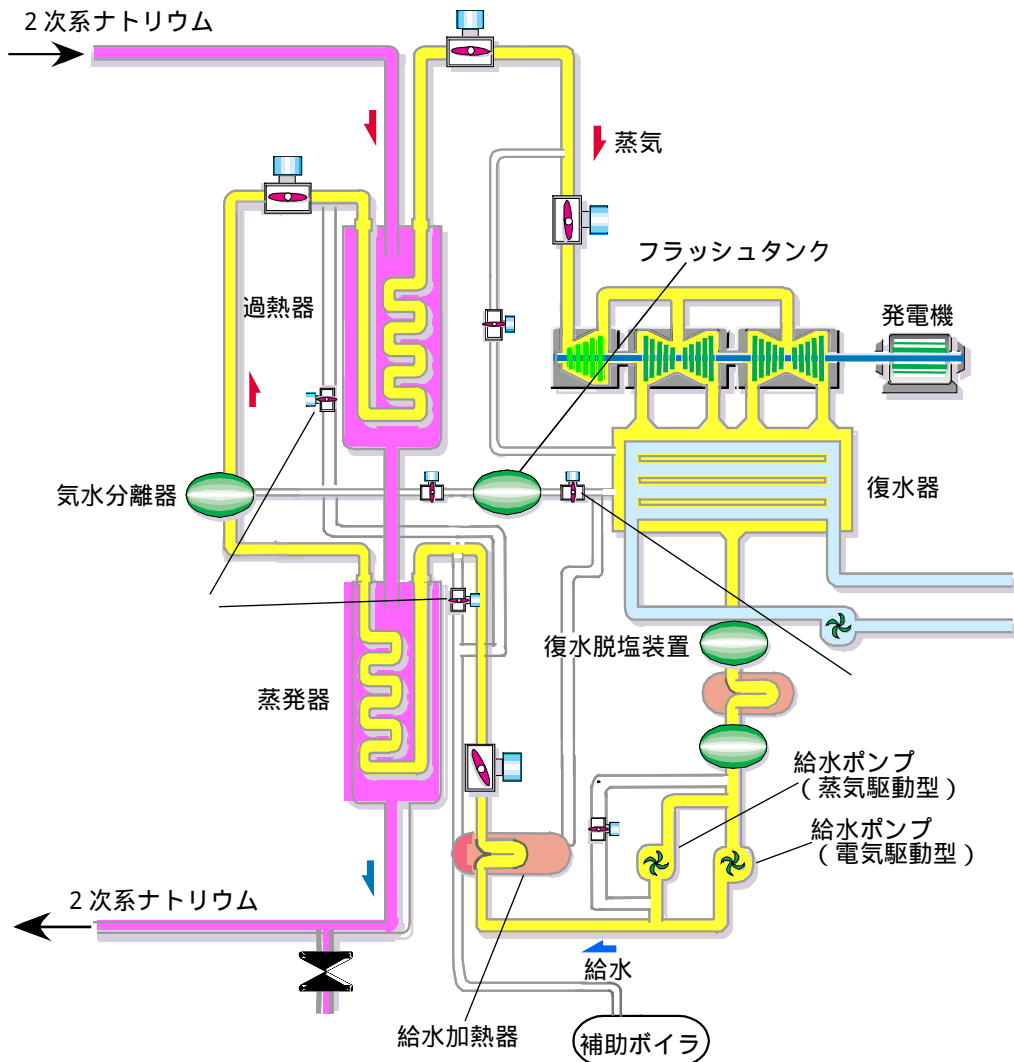
図 - 1 安全総点検に係る設備改善について (水蒸気系及びタービン設備の改善)
