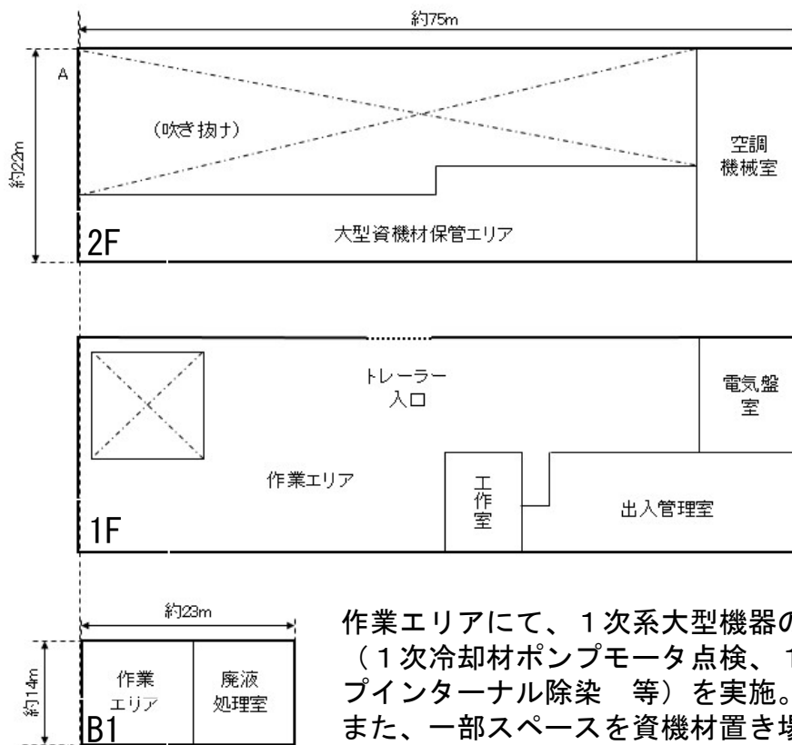
保守点検建屋概略図 平面図 (案)
