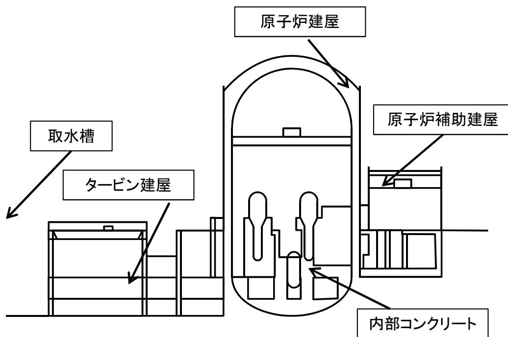
評価対象のコンクリート構造物
