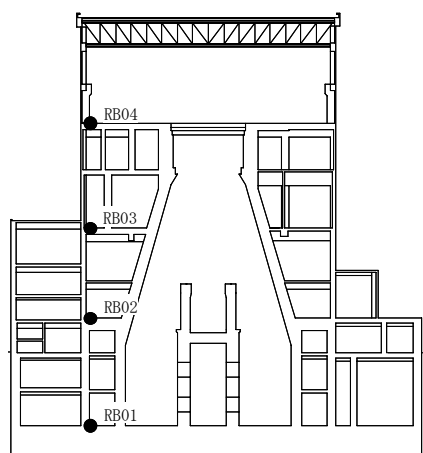
地震計配置(原子炉建屋)
