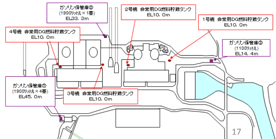
消防ポンプ・空冷式非常用DG用燃料の配置
